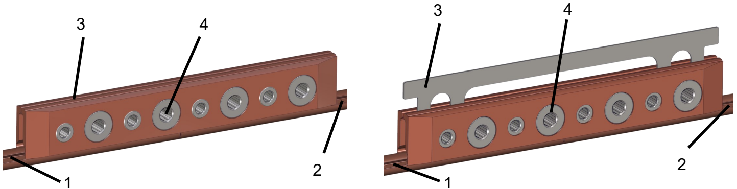
A Stossklemme für Fahrdrabtkerbe Typ AC, Fahrdrabtkerbe 5.51 - 5.60 mm
